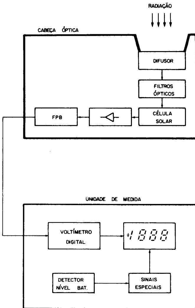
FIG.1 - DIAGRAMA EM BLOCOS DA CABEÇA ÓPTICA E DA UNIDADE DE MEDIDA
