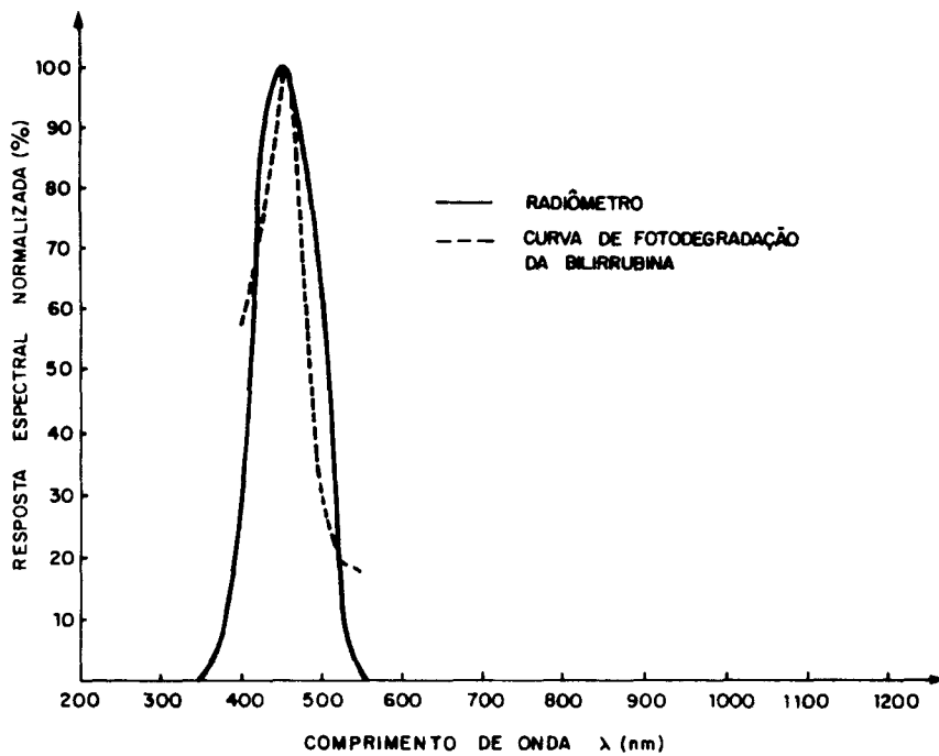
FIG. 2 - RESPOSTA ESPECTRAL DO RADIÔMETRO COMPARADA COM A CURVA PROPOSTA POR LANNING ET AL (1972) PARA A FOTODEGRADAÇÃO DA BILIRRUBINA .
